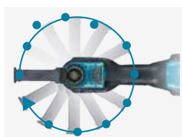
多角度設定刀片 0°–360° 共12個角度位置設置刀片
