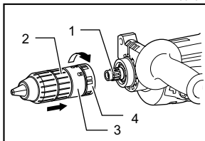
1. 主轴 2. 快换式钻机夹盘 3. 转换套指示线 4. 转换套
