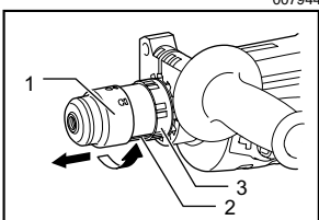
1. SDS-plus 的快换式夹盘 2. 转换套指示线 3. 转换套
