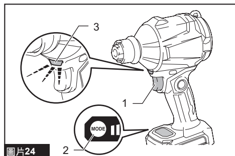
圖片24 ▶ 1. 開關扳機 2. 風量調整按鈕 3. 燈
