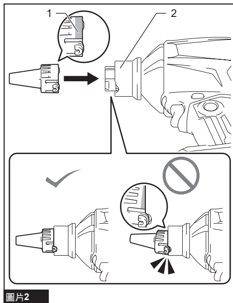
圖片2 ► 1. 拋光表面 2. 鎖緊套筒
