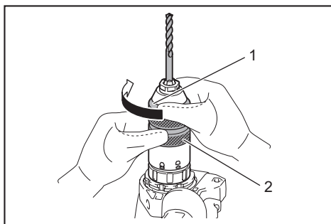
► 1. 套筒 2. 擋圈
