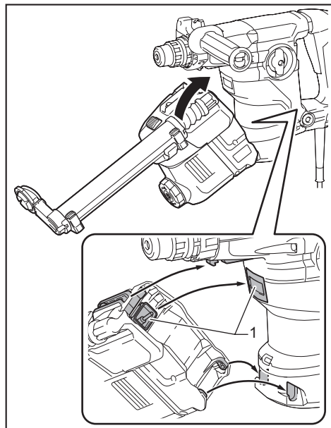
► 1. 空氣導管
