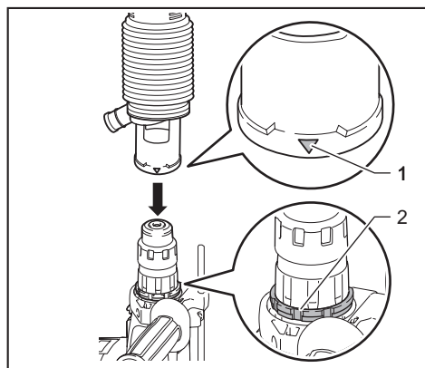
► 1. △ 符號 2. 溝槽
