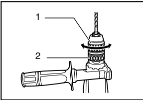
1. 套管 2. 卡盘环
