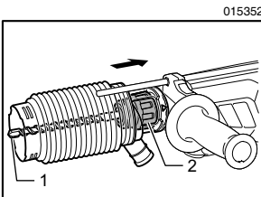
1. 钻头 2. 卡盘壳
