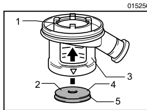
1. 内缘 2. 平坦侧 3. 装置 4. 盖 5. 凹槽
