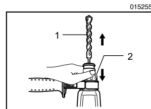
1. 钻头 2. 卡盘壳
