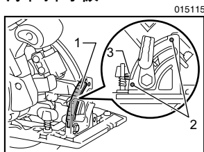
1. 斜导板 2. 螺丝 3. 导板
