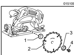
1. 内法兰盘 2. 锯片 3. 外法兰盘 4. 六角螺栓
