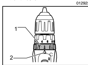
1. 动作模式切换环 2. 箭头
