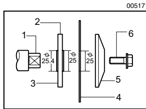
1. 安装轴 2. 内法兰盘 3. 25.4 毫米标记 4. 金刚石砂轮 5. 外法兰盘 6. 六角螺栓
